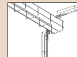
Skjøtefestet kan brukes til vertikal eller horisontal montering av minitrådstiger på trådstiger og kabelstiger.
