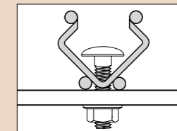
B30-D kan monteres med Skruesett B13, alternativt skrue med stort hode, egnet for tre, betong mm.
